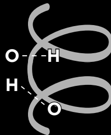
Création d'une nouvelle liaison hydrogène en séchant et en coiffant les cheveux (kératine bêta)
