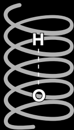
Liaison hydrogène avant le coiffage (kératine alpha)
