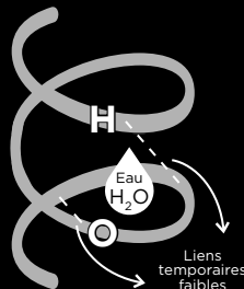
Liaison hydrogène brisée par l'eau
